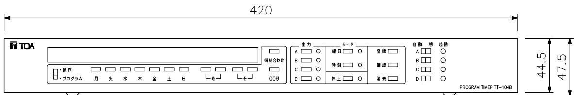
正面図
