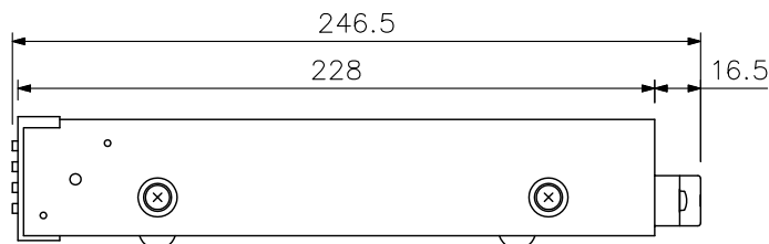
側面図
