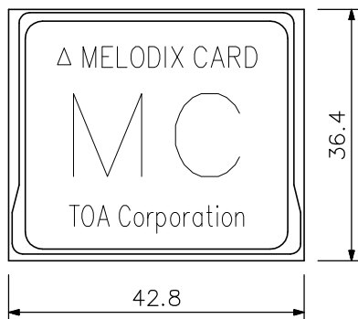
正面図
