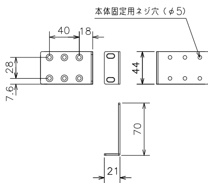
19インチラック固定用金具 (同梱)
