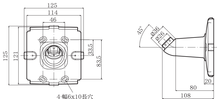
＜カメラ取付台寸法図＞(単位:mm)
