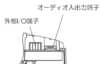
＜矢視B＞
