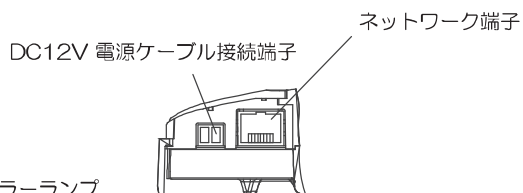
＜矢視A＞
