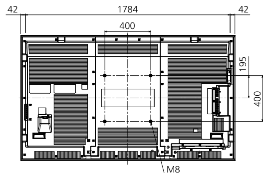
(注) この図面は縮尺ではありません。 単位：mm
