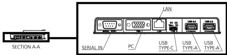
端子部拡大図 a
