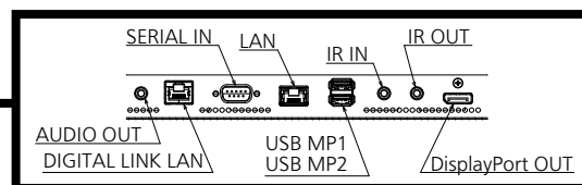
端子部拡大図 a
