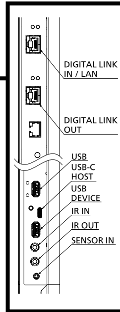
端子部拡大図b
